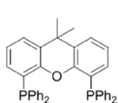
Xantphos
