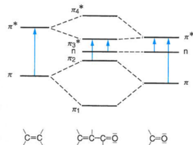
図 1.25 アルケンおよび飽和カルボニル化合物と比較した共役エノンの電子遷移エネルギー図
