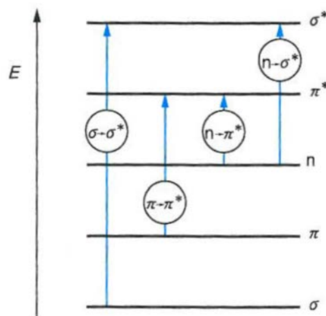
図 1.6 分子軌道と電子遷移
