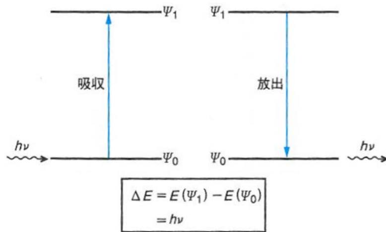
図 1.2 電子遷移および放射過程
