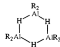
R = C 2 H 5 , (CH 3 ) 2 CHCH 2 など (8) (\text{R}_2\text{AlH})_3 の水素架橋三量体構造
